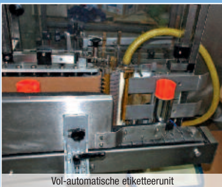
Vol-automatische etiketteerunit
